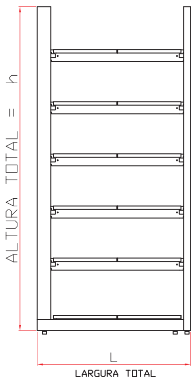
CORTE
